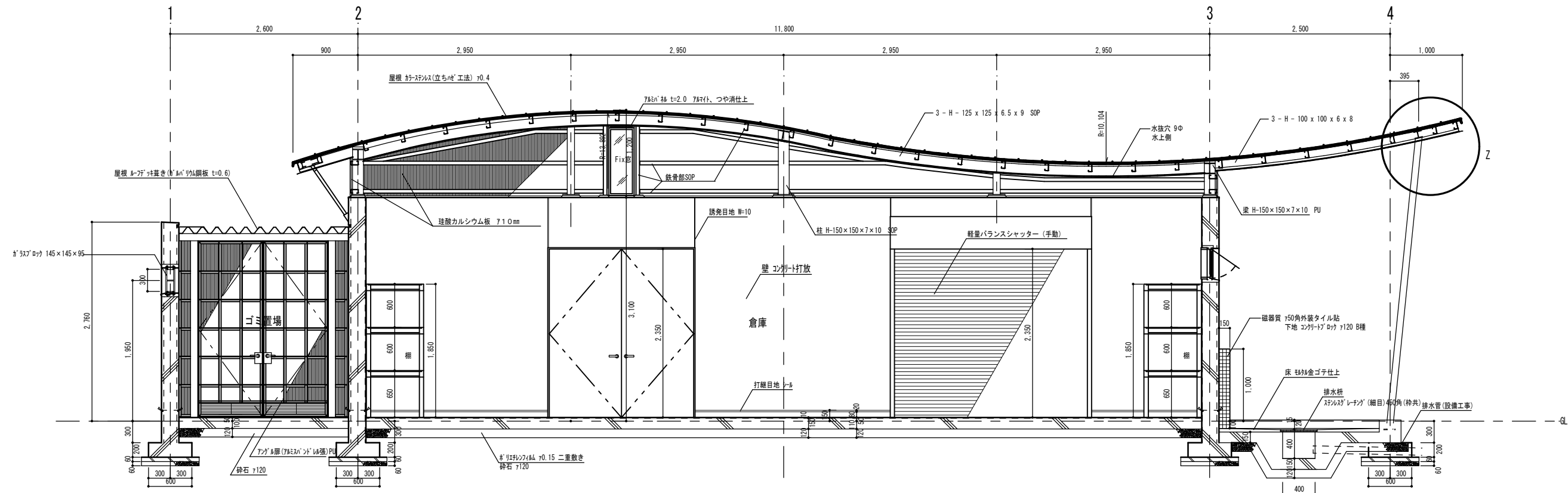
M部 断面図 1:30
