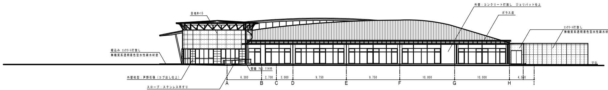
東立面図
