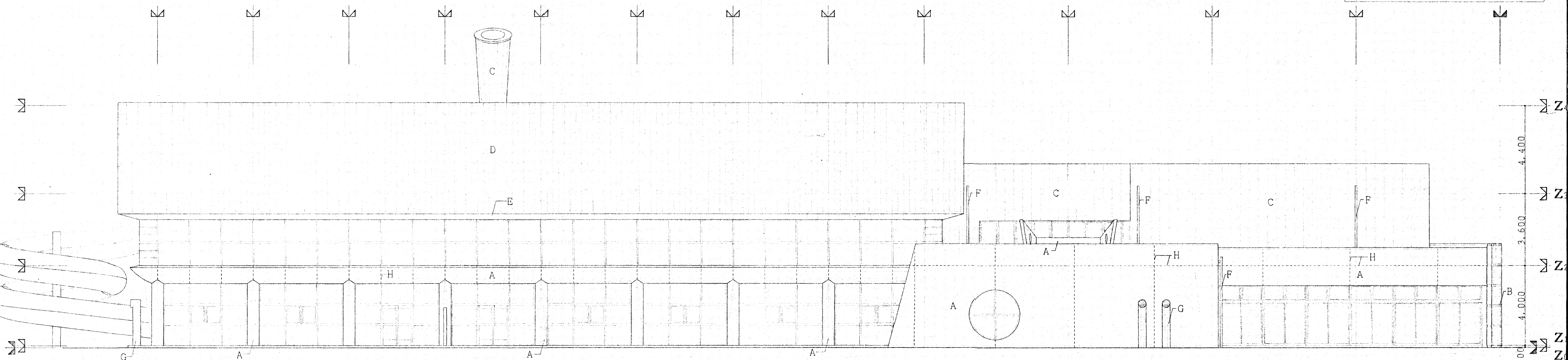
東側立面図 1/100
