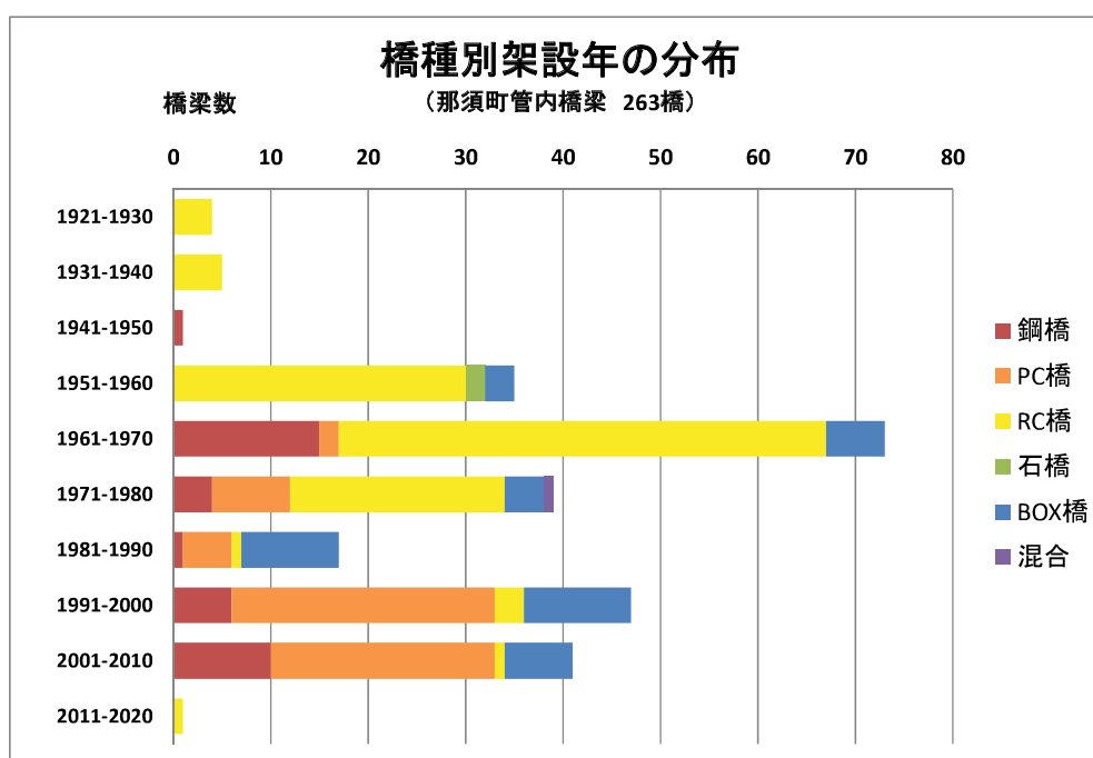
図 3.1.4 橋種架設年別の分布
