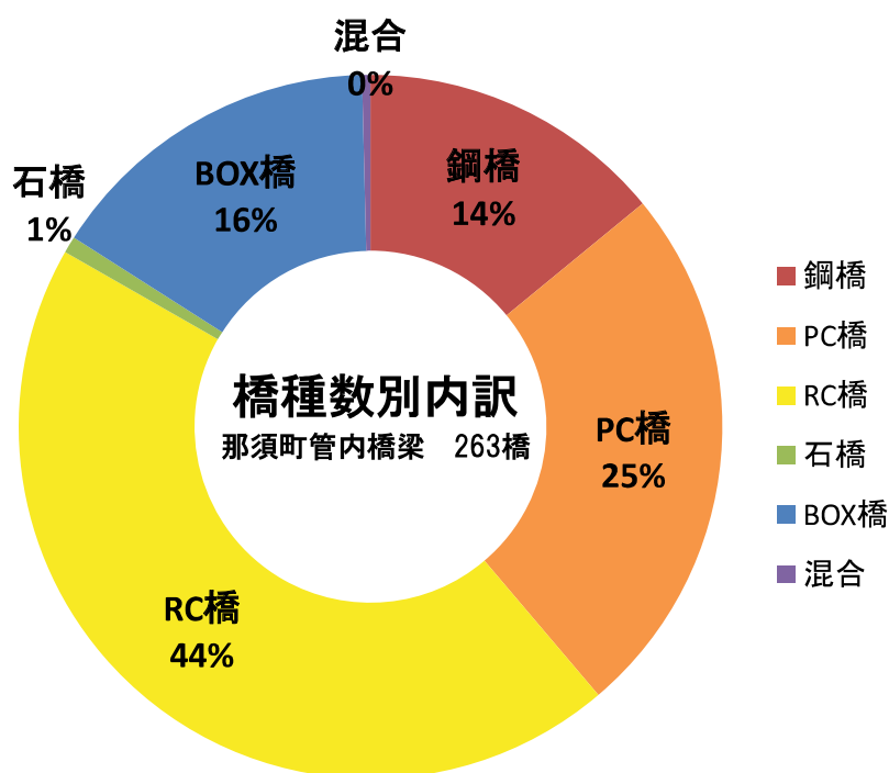
図 3.1.3 橋種別内訳
