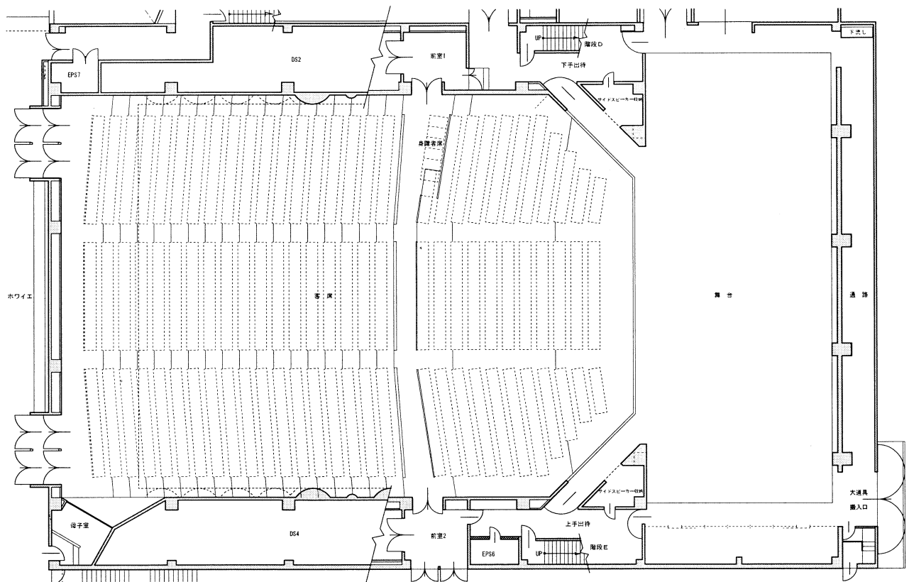
大ホール平面図【那須町文化センター】
